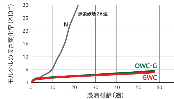
25g/L MgSO 4 溶液中での膨張率
