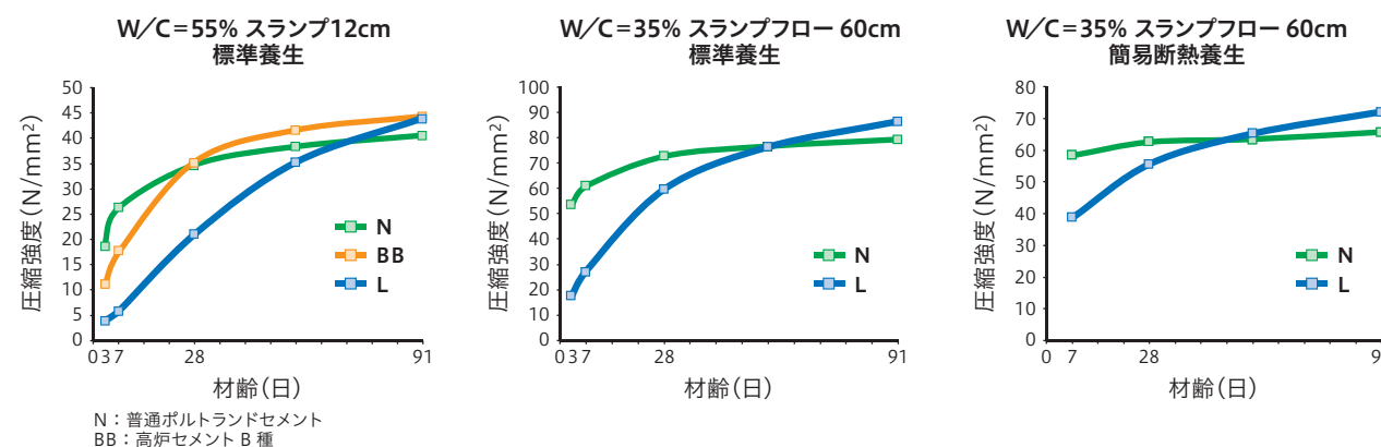
材齢と圧縮強度
