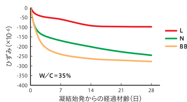
自己収縮ひずみ
