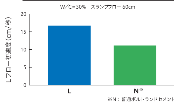
同一スランブフローでのLフロー初速度
