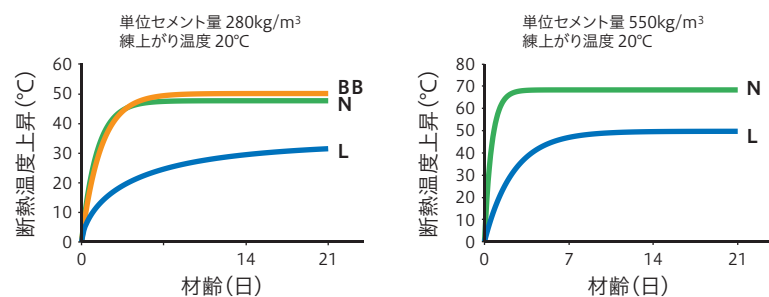
断熱温度上昇量
