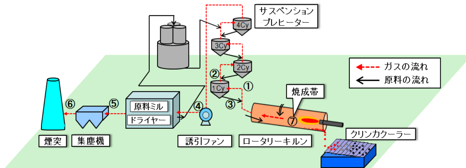
図 セメント製造工程の概略図
