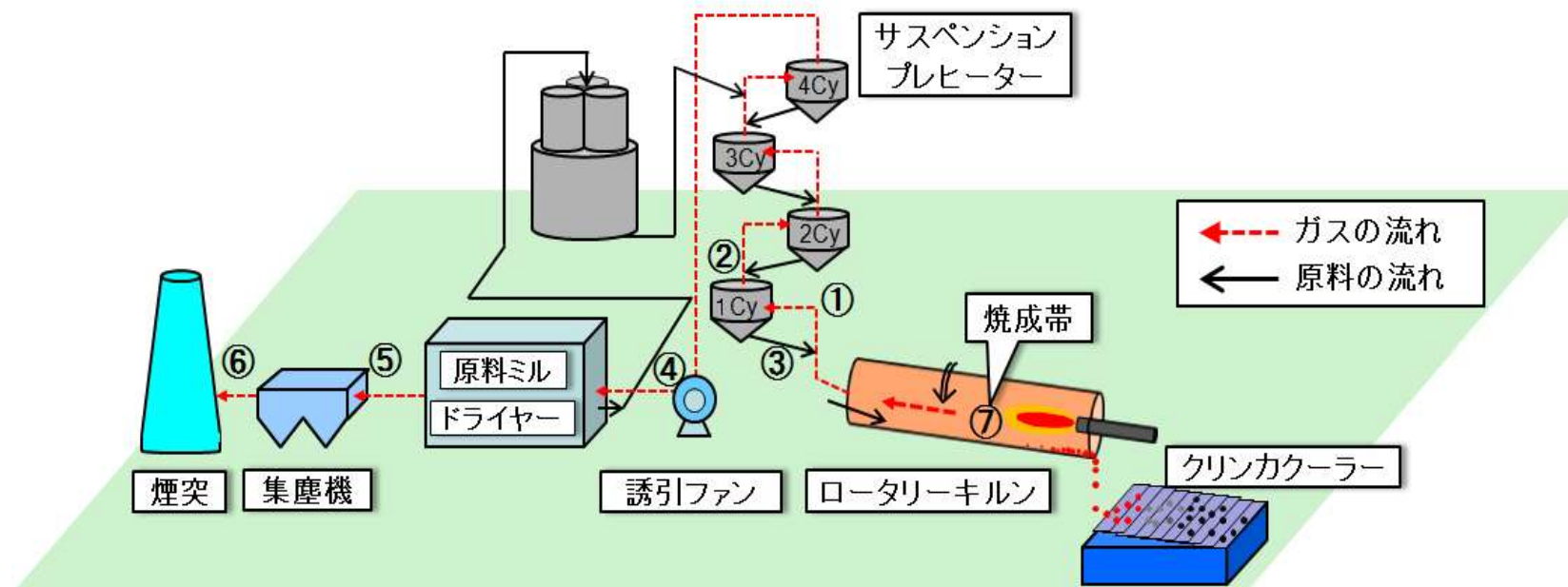
図 セメント製造工程の概略図
